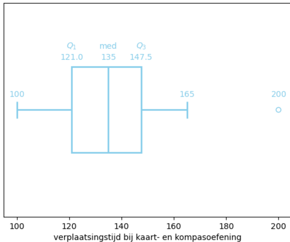
Boxplot van verplaatsingstijden bij kaart- en kompasoefening
